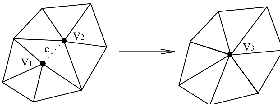
Рис. 3. Стягивание ребра
