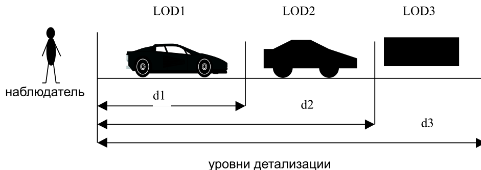
Рис. 6. Диапазоны LOD
