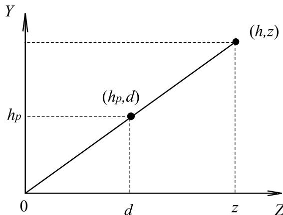
Рис. 15. Перспективная проекция
