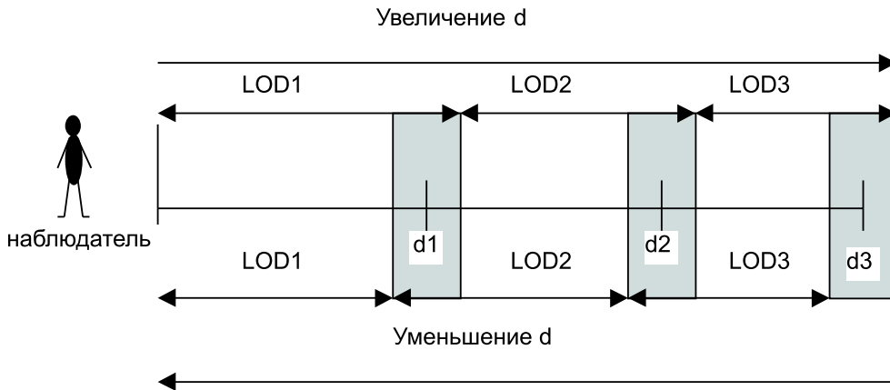
Рис. 7. Перекрытие диапазонов
