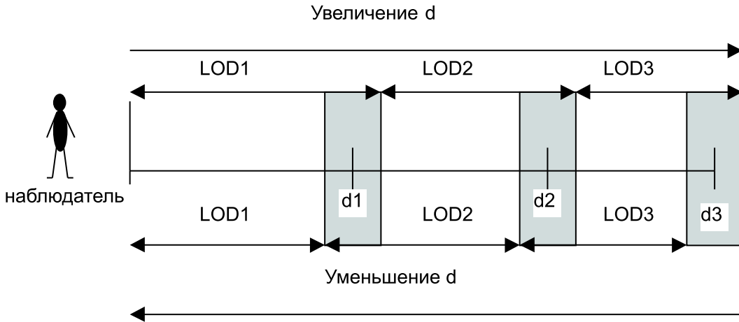
Рис. 8. Изменение площади проекции ограничивающего объема на картинную плоскость
